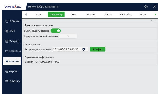
Рисунок 4.6. Меню настроек
